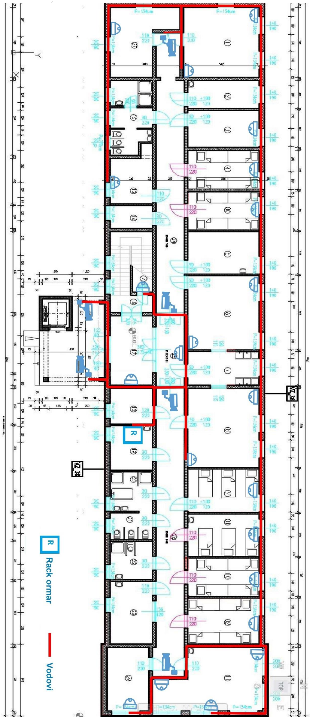
Slika 2. ZGRADA 2 – odjel VI - prizemlje (vodovi)
