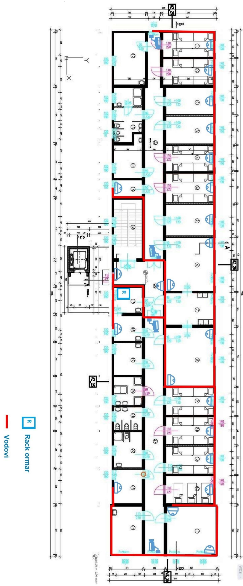
Slika 4. ZGRADA 2 – odjel IV - kat (vodovi)
