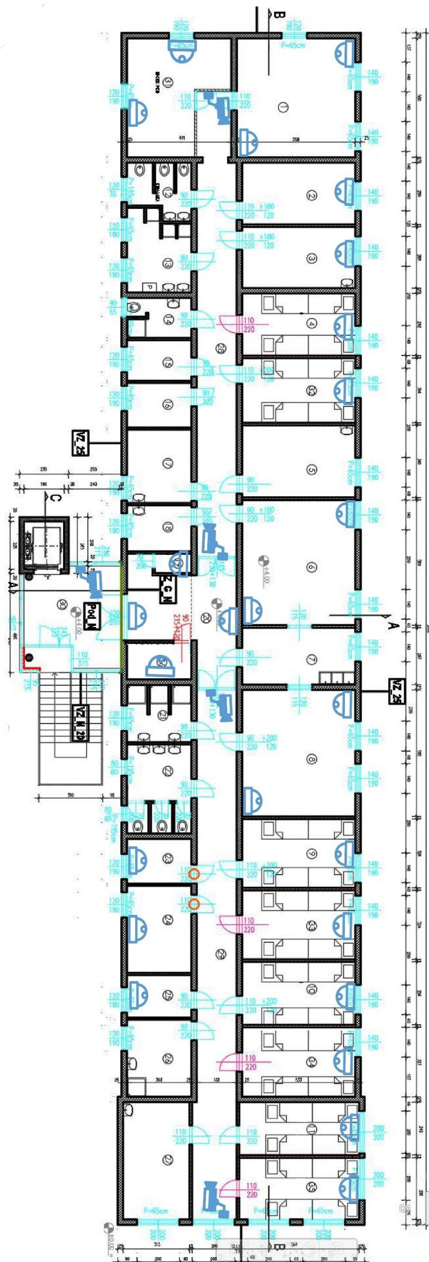
Slika 3. ZGRADA 3 – odjel XI – kat (raspored kamera)
