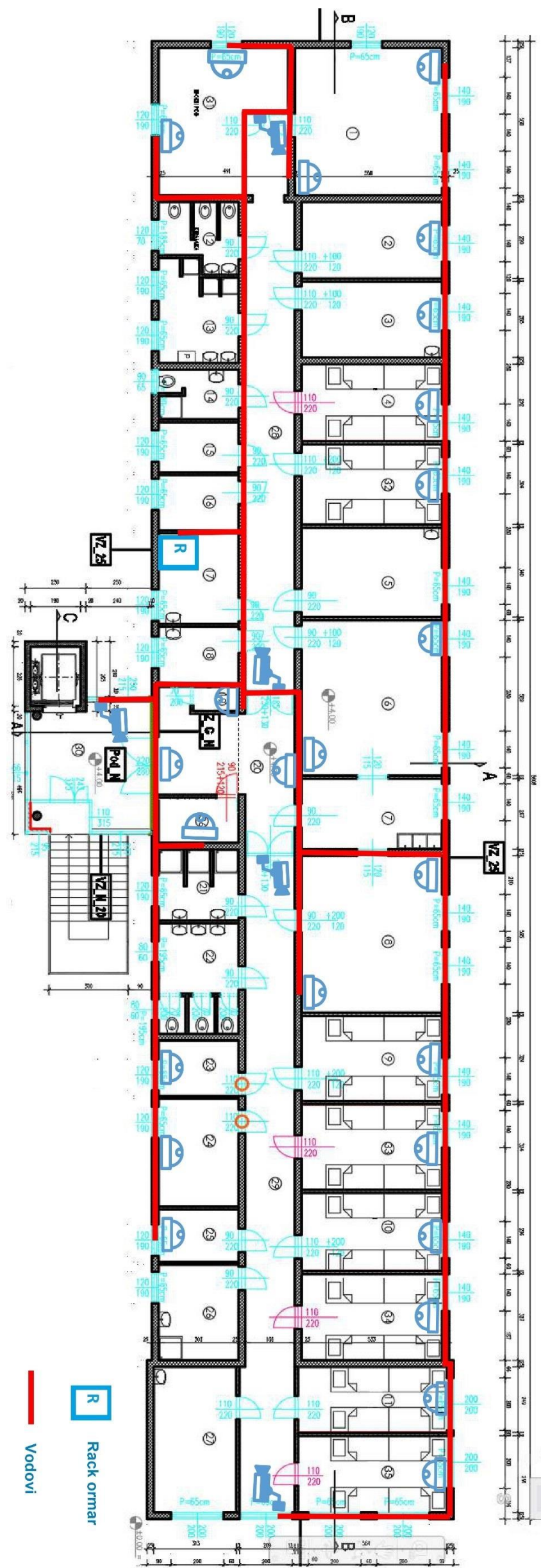
Slika 4. ZGRADA 3 – odjel XI – kat (vodovi)
