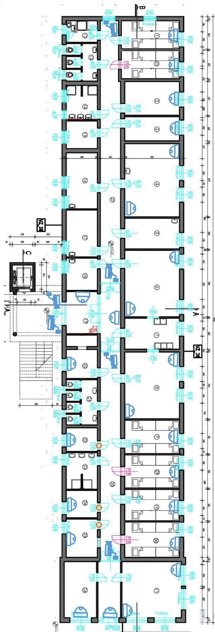
Slika 1. ZGRADA 3 – odjel V – prizemlje (raspored kamera)
