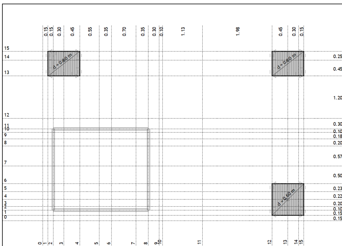
Nivo: temelji stupova [-0.90 m]
