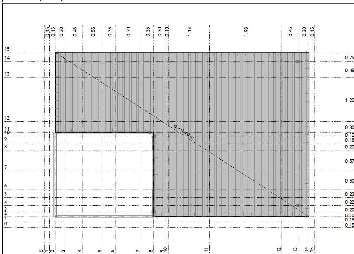
Nivo: 1. kat [3.97 m]
