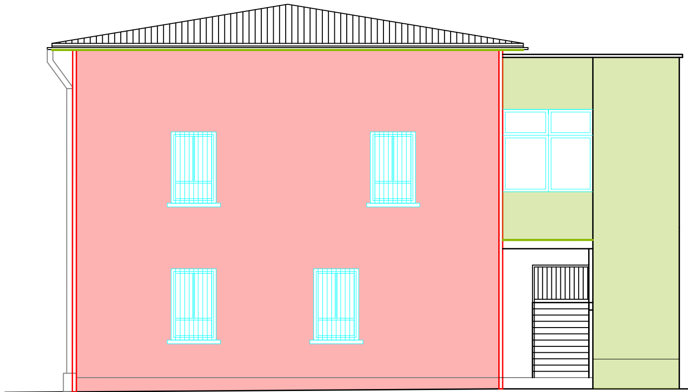
PROČELJE SJEVEROISTOK
