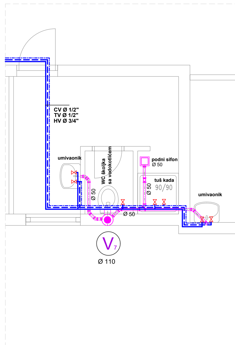
SANITARNI ČVOR - E
