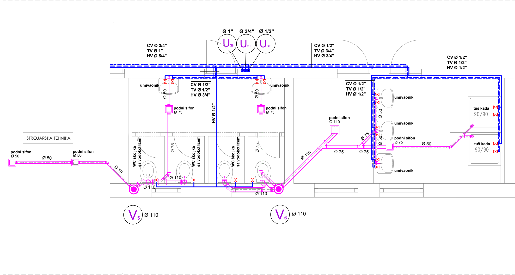
SANITARNI ČVOROV I - B
