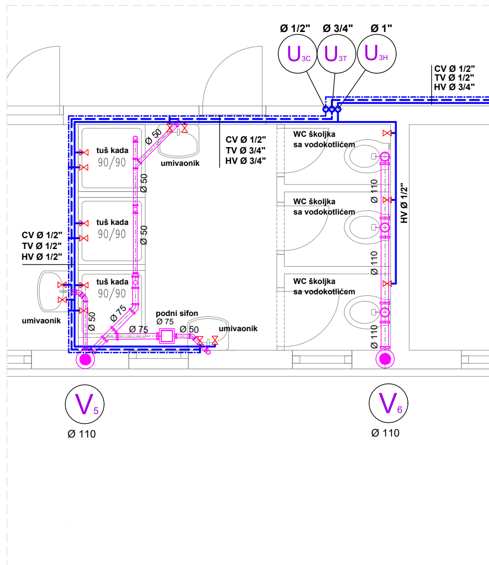
SANITARNI ČVOR - D
