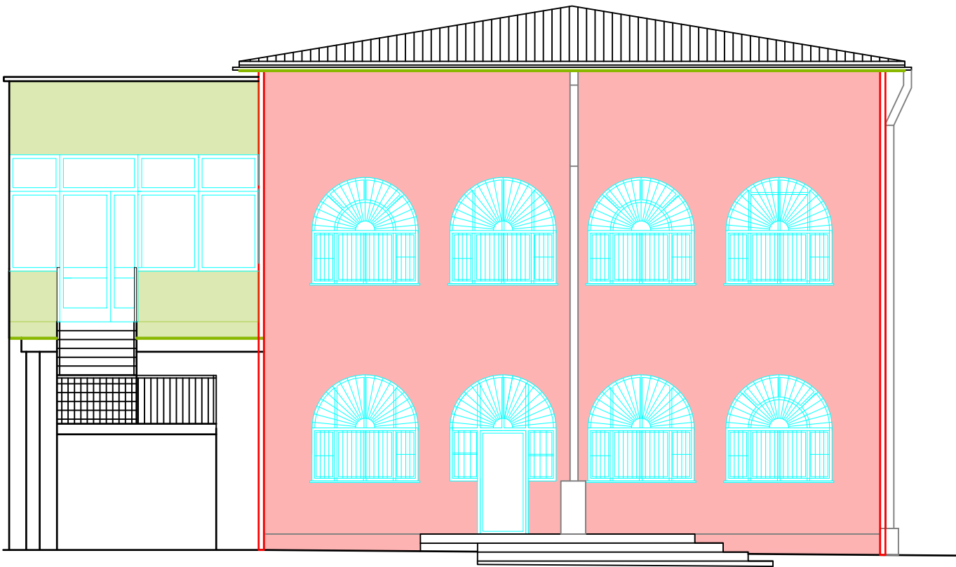
PROČELJE JUGOZAPAD
