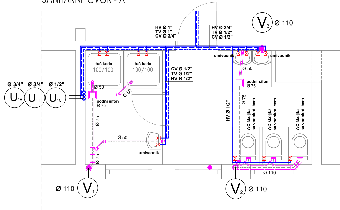
SANITARNI ČVOR - A
