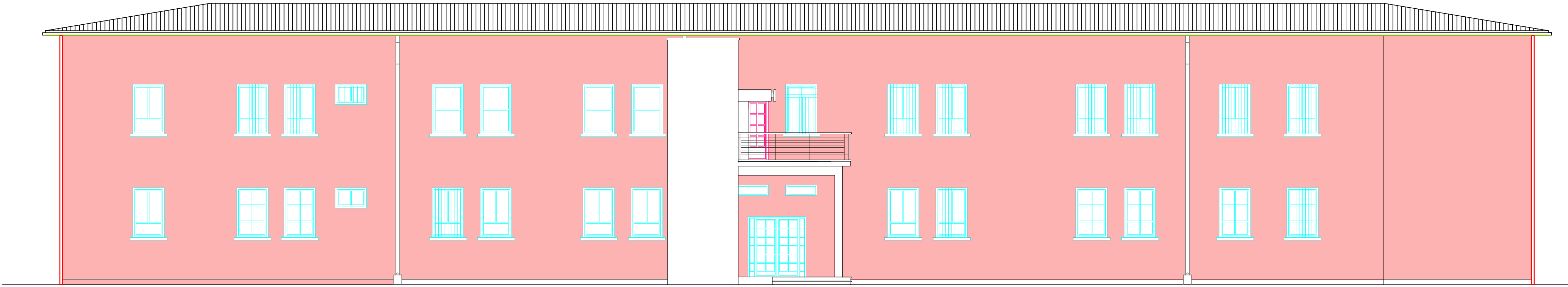
PROČELJE SJEVEROZAPAD
